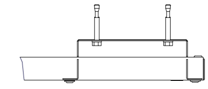
Particolare B scala 1 : 5
